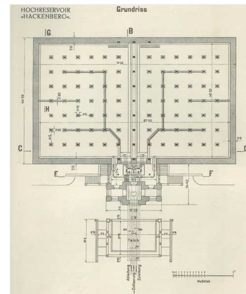
Grundriss des Wasserreservoir Hackenberg
