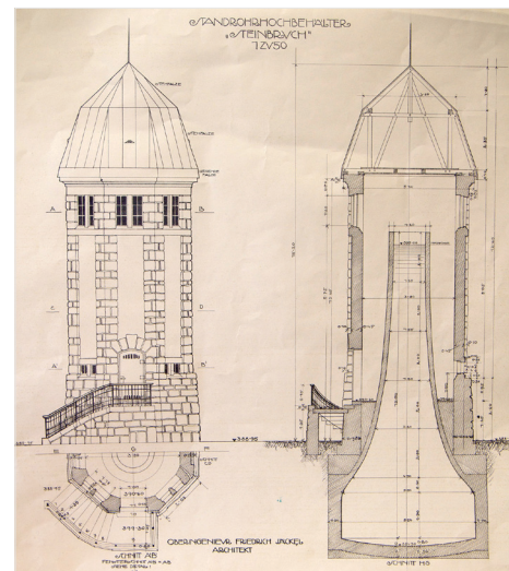
Standrohrbehälter „Steinbruch“ ident mit dem Bauwerk am Dreimarkstein
